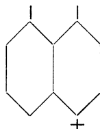
Dioxynaphtalin- sulfosäure S. D.R.P. 54116.
